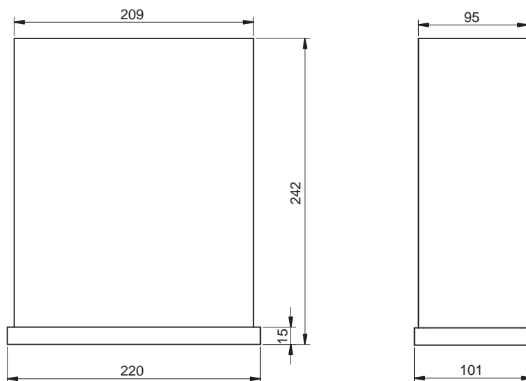
Схема внешних габаритов HMBK-10/ HMBK-35
